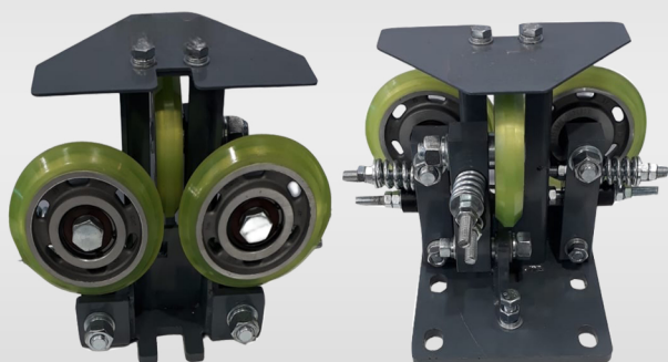
ROLLER GUIDE SHOE- Ø 125MM- SKG 4
